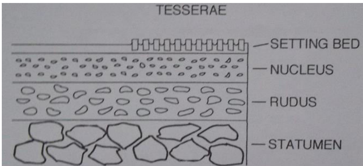
Obrázok 48: vrstvy podlahy, podľa Dunbabin 1999, obr. 288.
