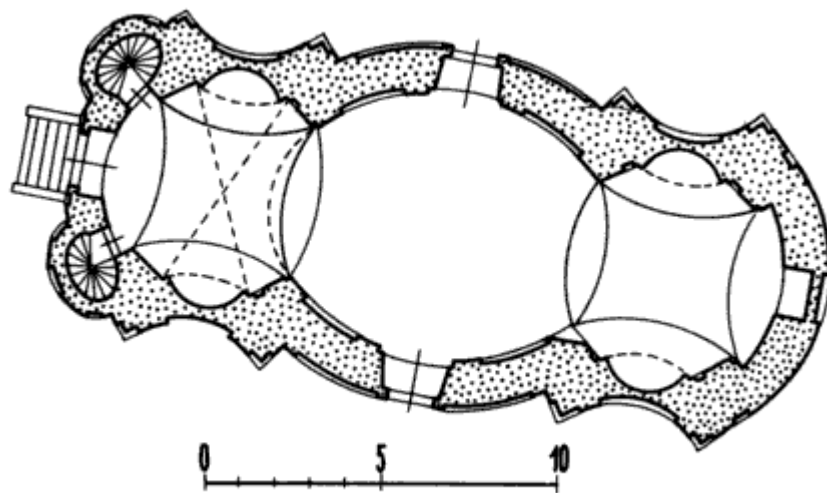
39. Odolena Voda, kostel sv. Klimenta. Půdorys.
