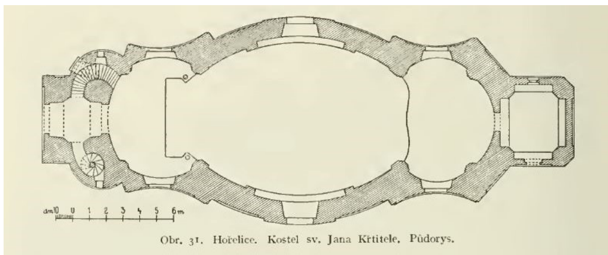
2. Rudná – Hořelice. Kostel Stěti sv. Jana Křtitele. Půdorys.
