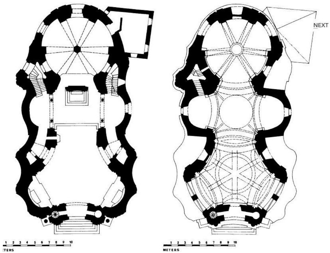
48. Aglie, kostel San Marta. Půdorys v rovině podlahy a v rovině kleneb.
