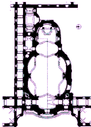
35. Verněřovice, kostel sv. Michaela. Půdorys.
