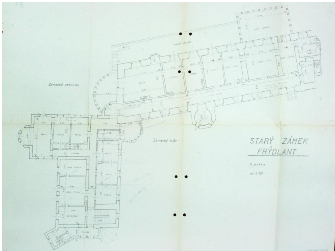
12. Frýdlant, Dolní zámek, půdorys druhého patra
