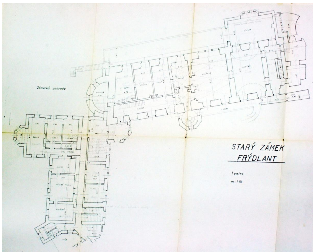
11. Frýdlant, Dolní zámek, půdorys prvního patra
