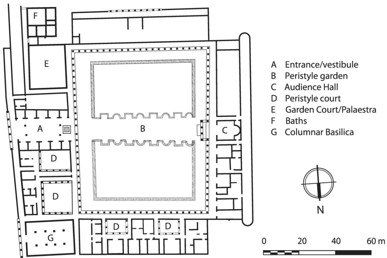
Obr. 8: Rekonstrukce tzv. Fishbourne Palace ve Velké Británii (nahore) a jeho půdorys (dole) (podle Yegül – Favro 2019, obr. 93).
