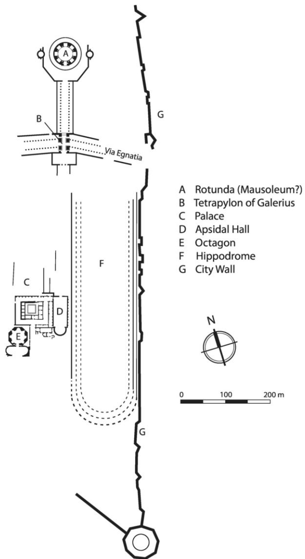
Obr. 37: Detail dochované části palácového komplexu a přidruženého hippodromu v Thessalonické (podle Ward-Perkins 1970, obr. 304).
