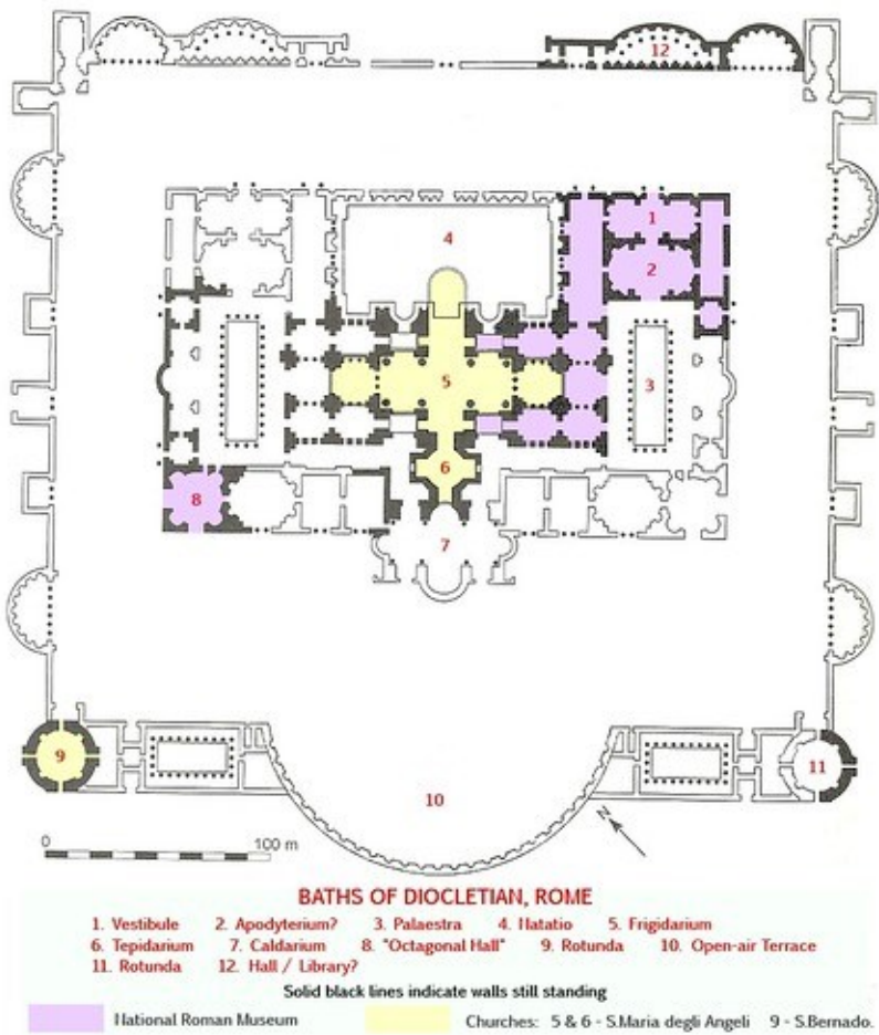
Obr. 36: Půdorys Diocletianových lázní v Římě se zvýrazněnými prostory dnešního muzea (fialově) a baziliky (žlutě) (podle Fletcher 2013, obr. 1174).
