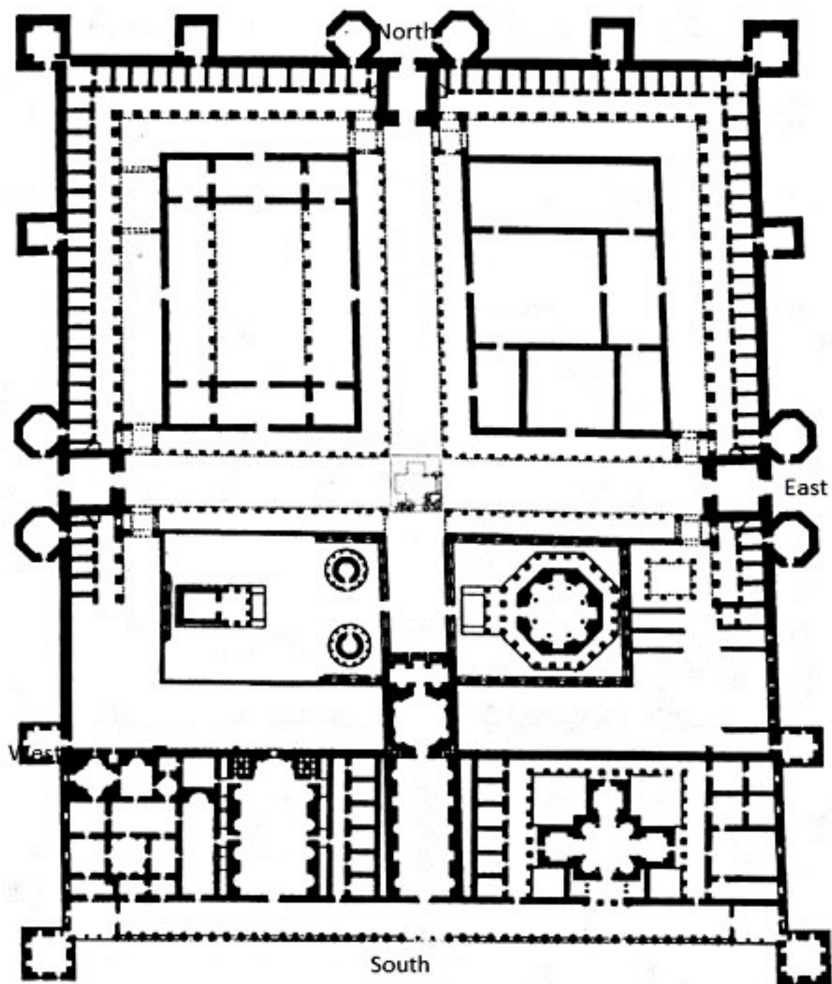
Obr. 27: Půdorys Diocletianova paláce ve Spalatu (podle Ward-Perkins 1970, obr. 308).
