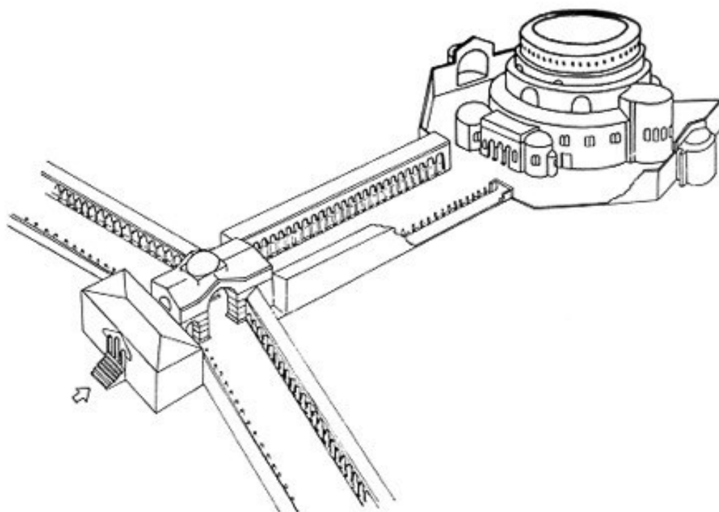
Obr. 45: Rekonstrukce Galeriova mauzolea v Thessalonické, portikové cesty a Galeriova triumfálního oblouku na via Egnatia (podle Ward-Perkins 1970, obr. 304).
