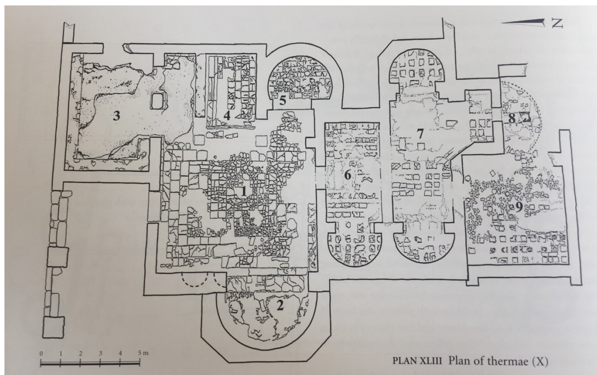
Obr. 35: Půdorys lázní ve Felix Romulianě (podle Popović 2011, obr. 43).
