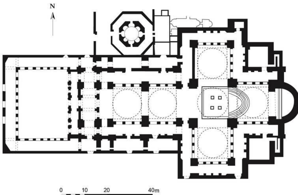
Obr. 54: Půdorys Konstantinova chrámu sv. Apoštolů s přidruženým císařským mauzoleem (Apostoleionem) (podle Johnson 2020, obr. 3).
