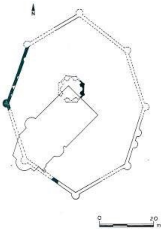
Obr. 48: Půdorys Maxentiova mauzolea se zvýrazněnými zachovanými částmi (tučně) a půdorysem dnešního kostela (podle Mikulka 2008, obr. 112).
