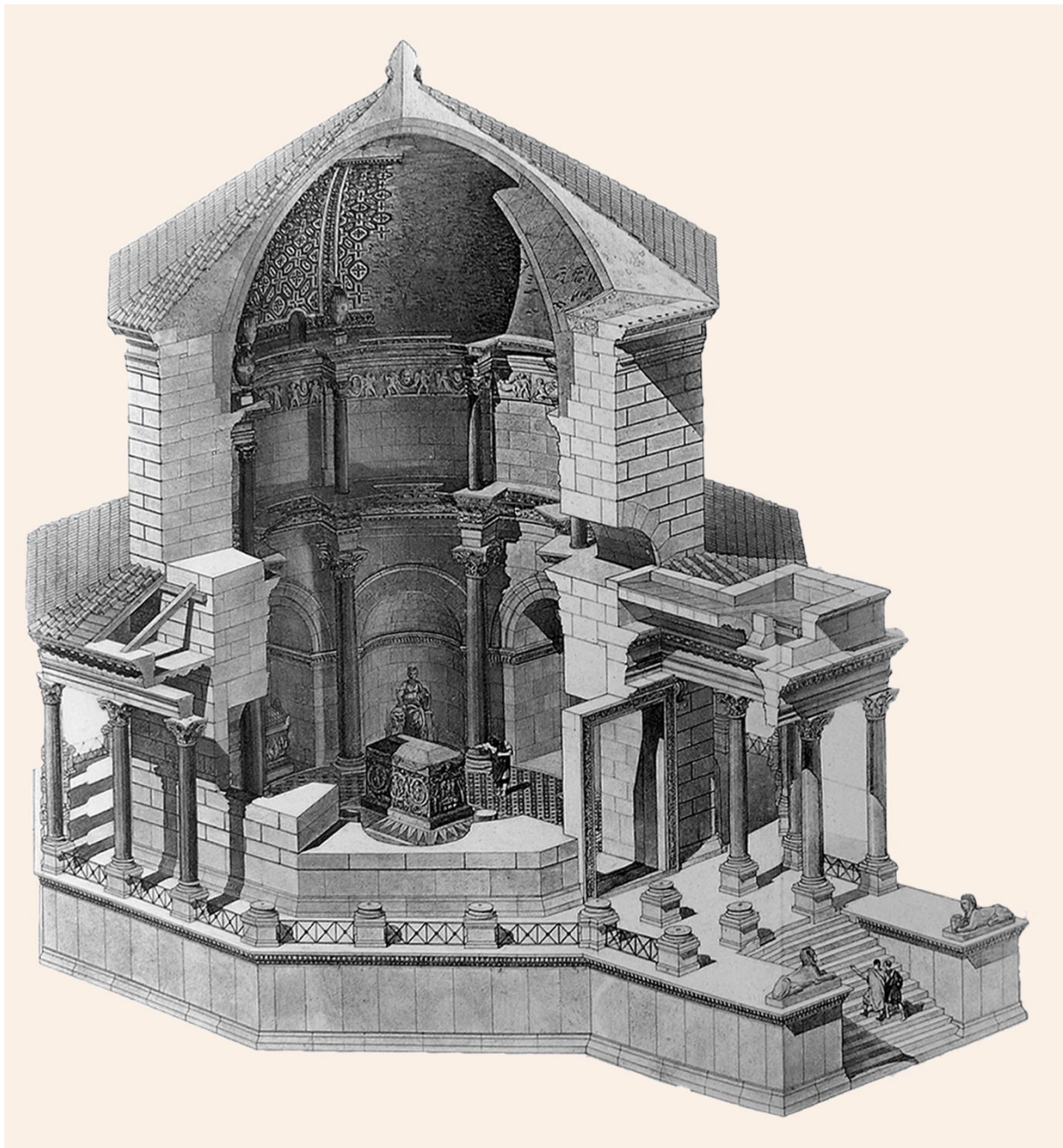
Obr. 41: Ideální rekonstrukce mauzolea se sarkofágem umístěným v celle (podle Hébrard 1920, obr. 13).
