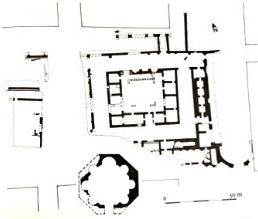
Obr. 32: Detail osmiúhelníkové místnosti s nikami v Thessaloníkě (podle Ward-Perkins 1970, obr. 305).
