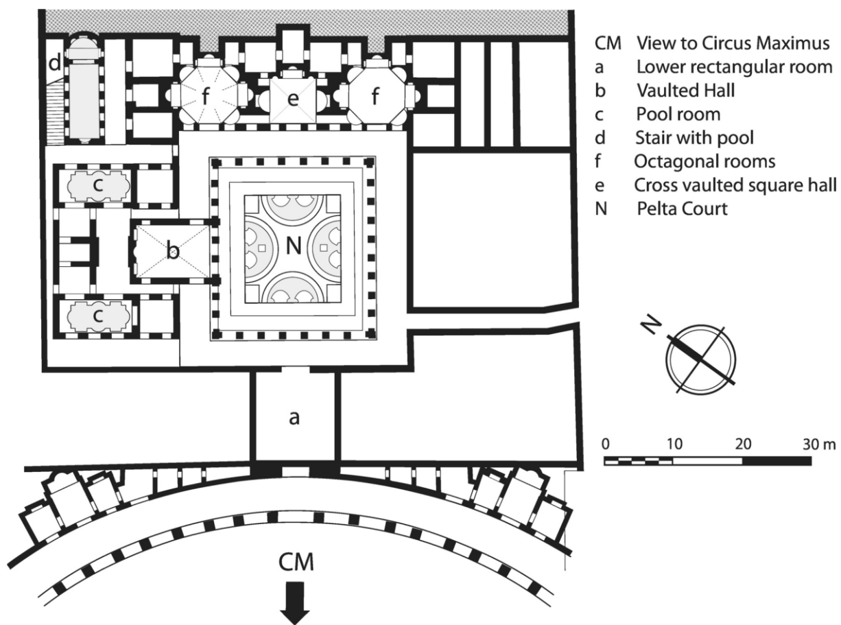
Obr. 26: Půdorys domu Flavia (podle Yegül – Favro 2019, obr. 58).
