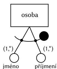
Obrázek 2.6: Příklad vizualizace schematické kategorie
