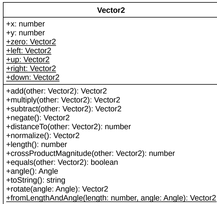
Obrázek 3.8: Diagram tříd – Vector2
