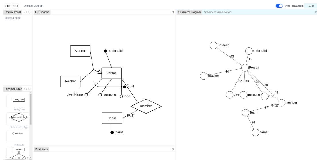
Obrázek 4.1: Ukázkou uživatelského rozhraní aplikace
