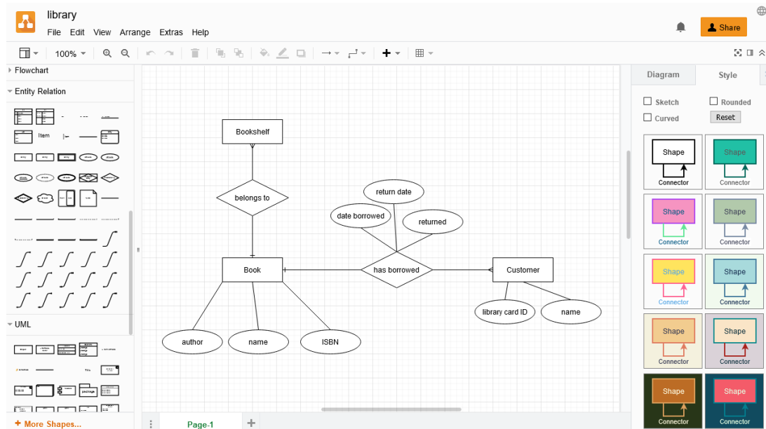
Obrázek 1.1: Tvorbba ER diagramu v aplikaci diagrams.net
