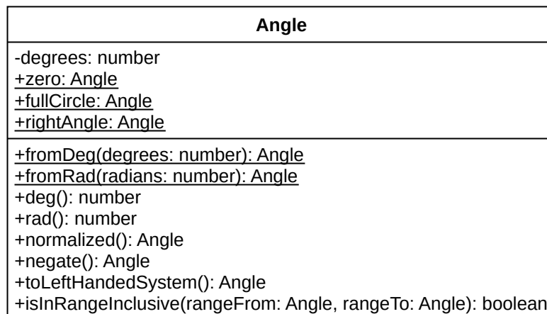
Obrázek 3.9: Diagram tříd – Angle
