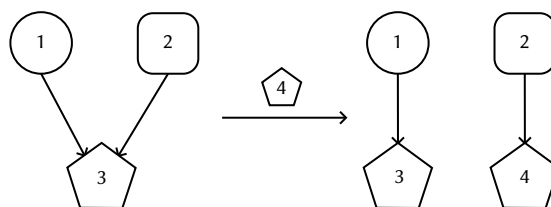
Obrázek 3.4: Ukázka problému immutability a referencí
