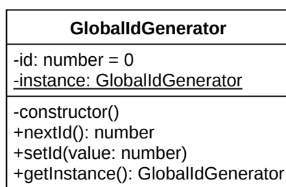
Obrázek 3.11: Diagram tříd – GlobalIdGenerator
