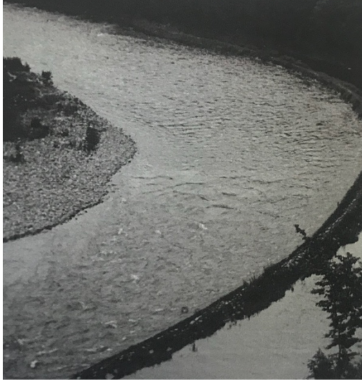
Ukázka vorařské navigace na SOUSÚ a na Pískách. Stejně navigace stály i na jiných místech toku. Navigace na Pískách je tak dokonale postavena, že stojí dodnes. Zdroj: Kronika osady Dakota 1926-2016.
