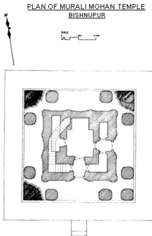
Obrázek 30: Plán chrámu Muralí Mohan
