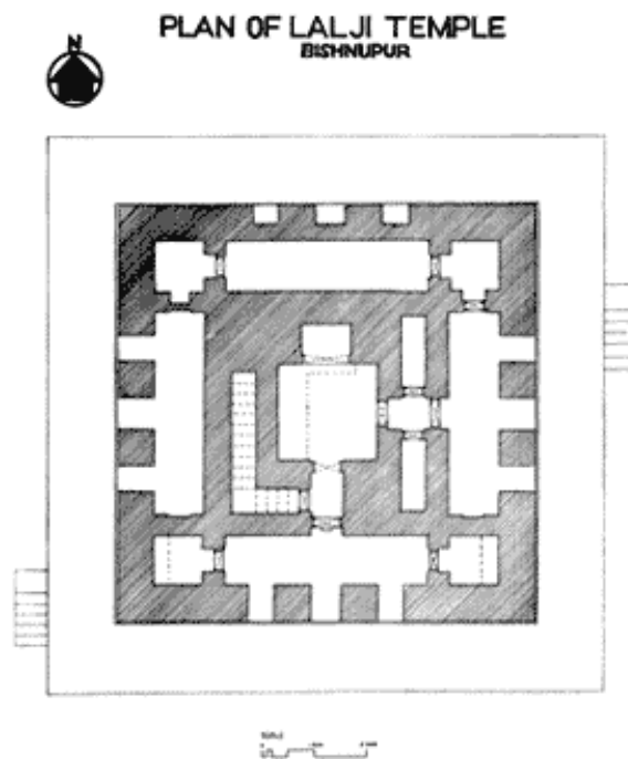
Obrázek 28: Plán chrámu Láldži
