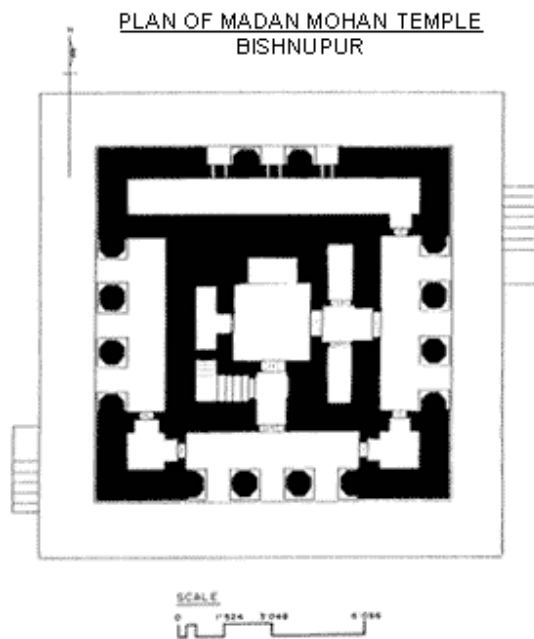
Obrázek 34: Plán chrámu Madan Mohan
