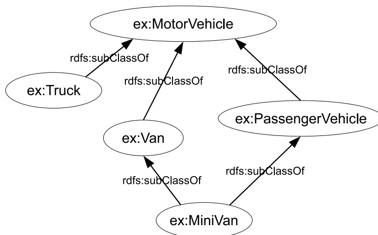
Obrázek 2.7: Příklad hierarchie tříd v RDF: A Vehicle Class Hierarchy Příklad pochází z dokumentu RDF Primer. http://www.w3.org/TR/rdf-primer/
