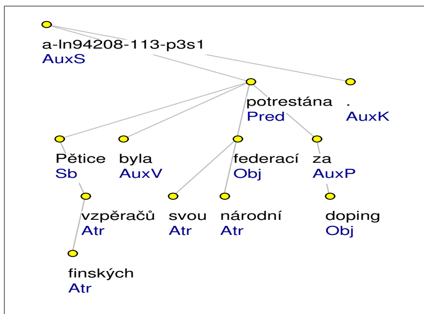
Obrázek 4.2: Příklad anotace na analytické rovině Podrobný popis obrázku je v sekci 4.1.4.
