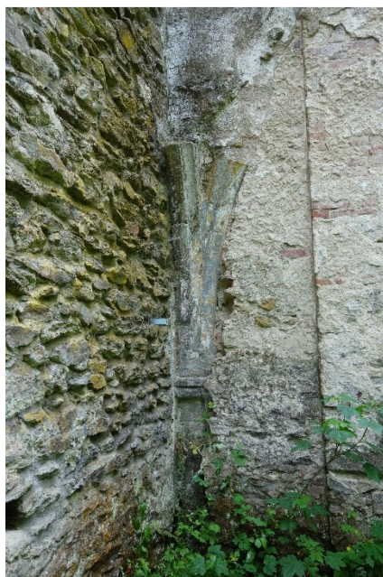
12. Pivoň, severní část presbytáře z exteriéru, výběh diagonálního a přízedního žebra, po 1230 nebo po 1260, pohled od severovýchodu
