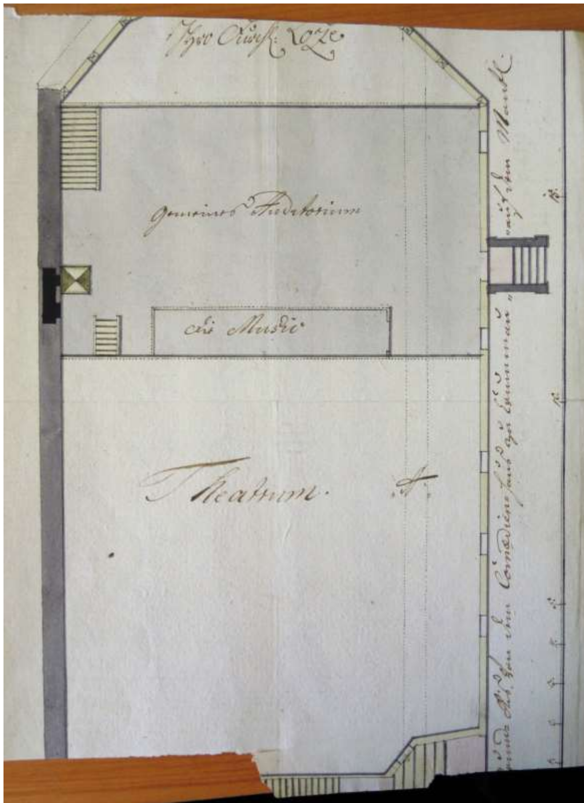
5. Plán starého zámeckého divadla v Českém Krumlově s návrhem úprav z roku 1760. SOA v Třeboni, pobočka Český Krumlov – Krumau: A 6B 2a (1744–1766).
