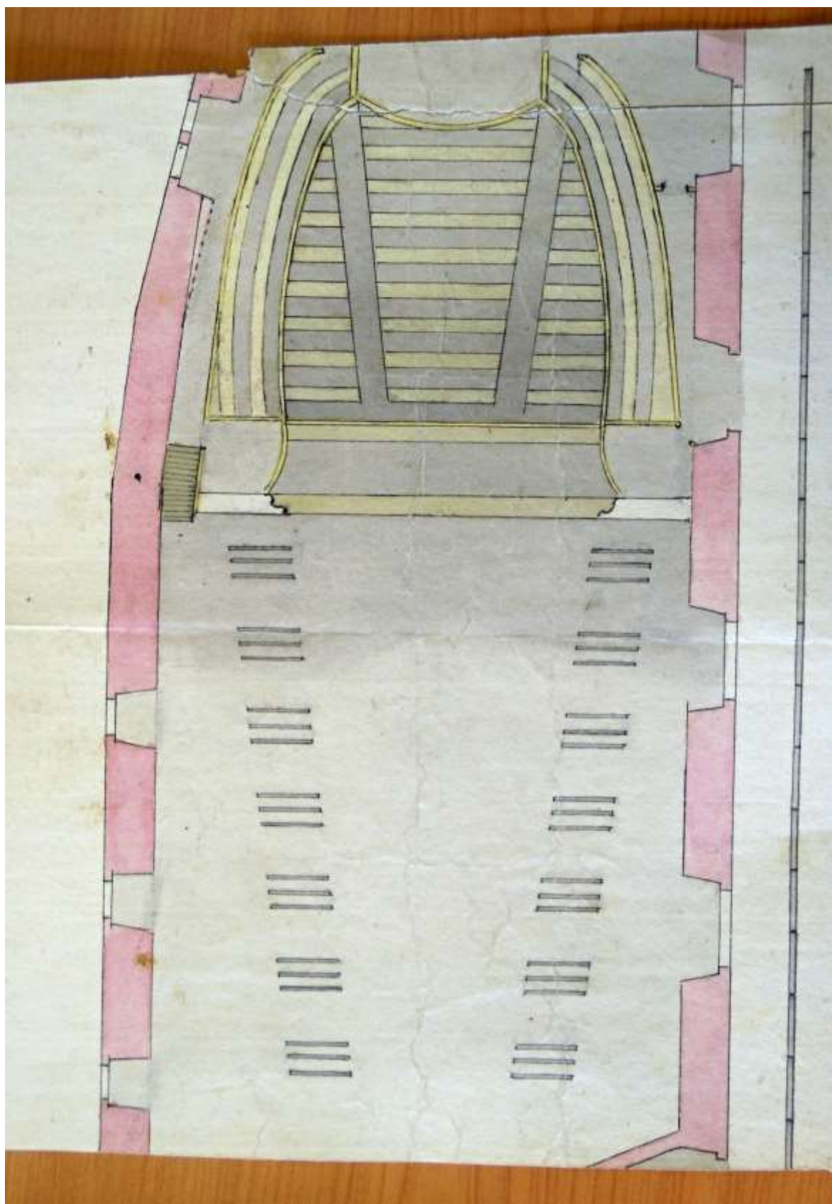
4. Návrh novostavby zámeckého divadla v Českém Krumlově z let 1760–1766. SOA v Třeboni, pobočka Český Krumlov – Krumau: A 6B 2a (1744–1766).
